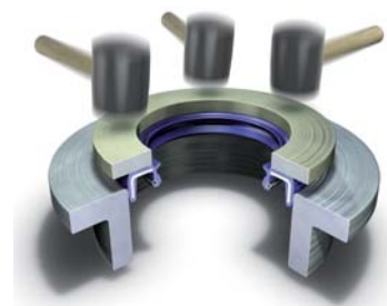
MONTAJE CON MAZA PERMITIDO
