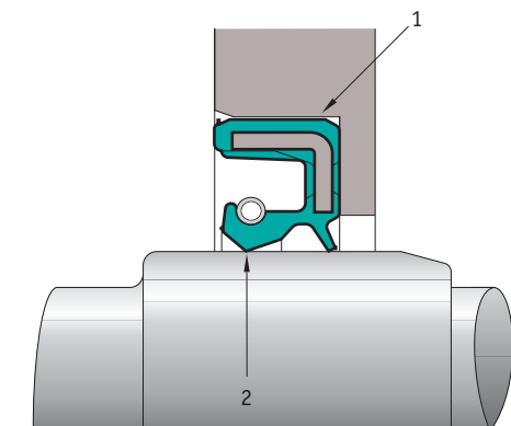
Retén radial estándar - configuración de montaje.
