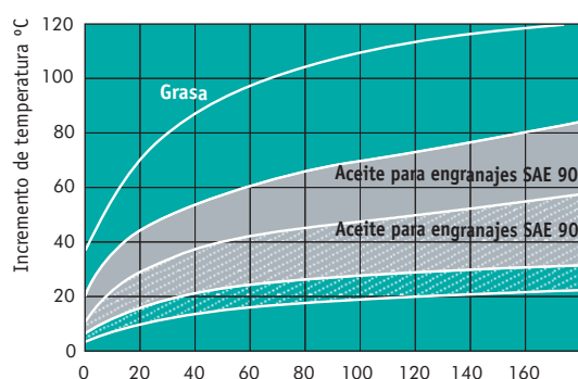
GRÁFICO 4. Incremento de temperatura en el punto a estanqueizar de un retén radial SIMMERRING® estanqueizando diferentes medios. Temperatura del baño de aceite 100° C. Número de revoluciones 3000 rpm.
