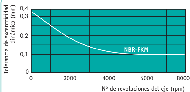
GRÁFICO 10. Tolerancia máxima de la excentricidad dinámica del eje en función del número de revoluciones
