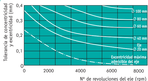
GRÁFICO 11. Tolerancia de concentricidad y excentricidad dinámica en función del número de revoluciones para la versión BASL
