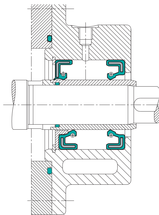
EJEMPLO DE MONTAJE 6: Obturación frente al vacío
